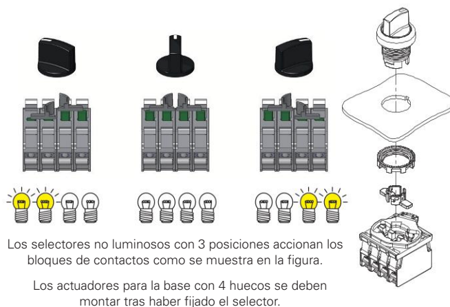
Base de fijación con 4 huecos
